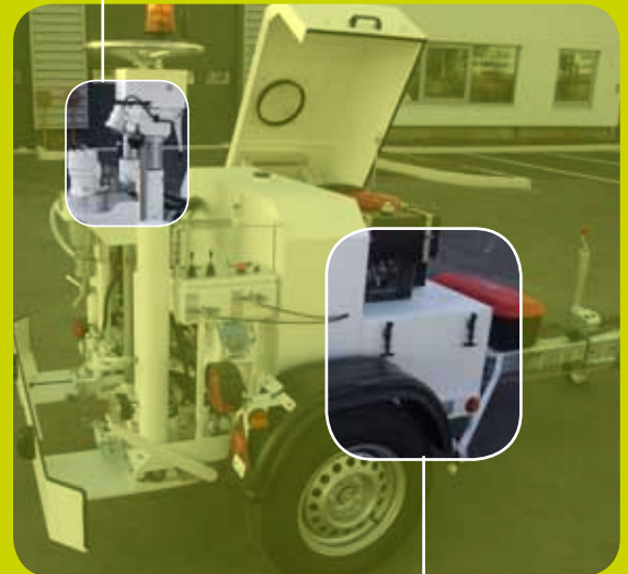
Coffre à outils - Machine livrée avec divers outils (clé à chaîne, pompe à graisse, clé plate,..)
